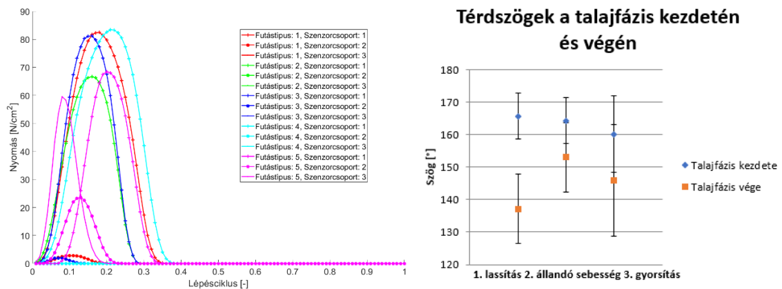
2. ábra. Nyomásértékek a 2. alany esetén (bal panel). Térdszögek (jobb panel).
