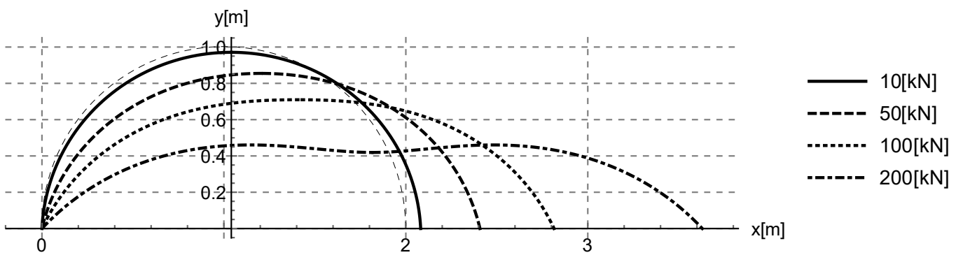
6. ábra. 10.4) kör keresztmetszetű rúdszerkezet deformálódott alakjai R = 1 [m], d = 50 [mm], E = 200 [GPa]
