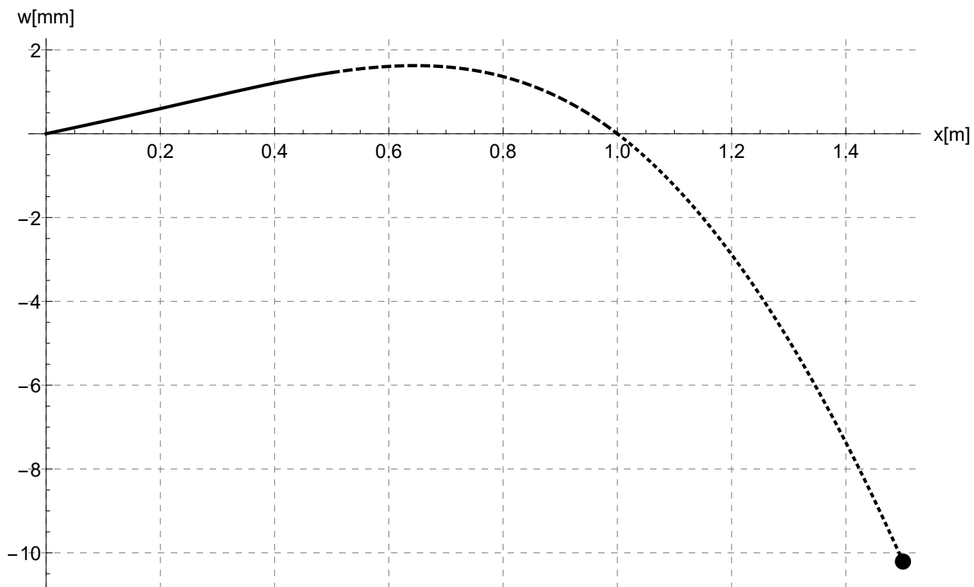
3. ábra. 10.2) lehajlás
