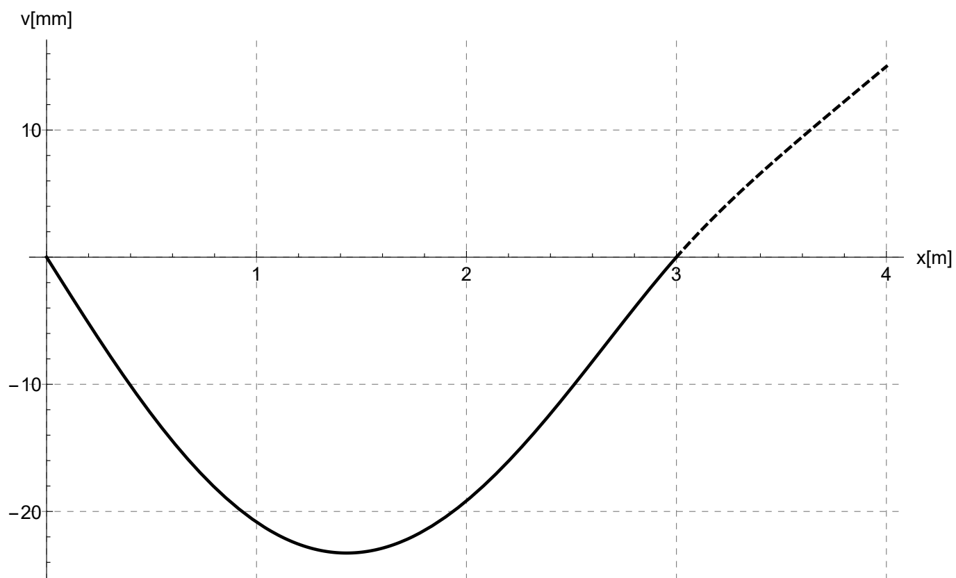
1. ábra. 10.1) lehajlás
