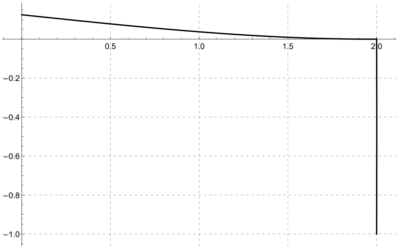
5. ábra. 10.3) deformálódott alak (10×-es nagyítás)
