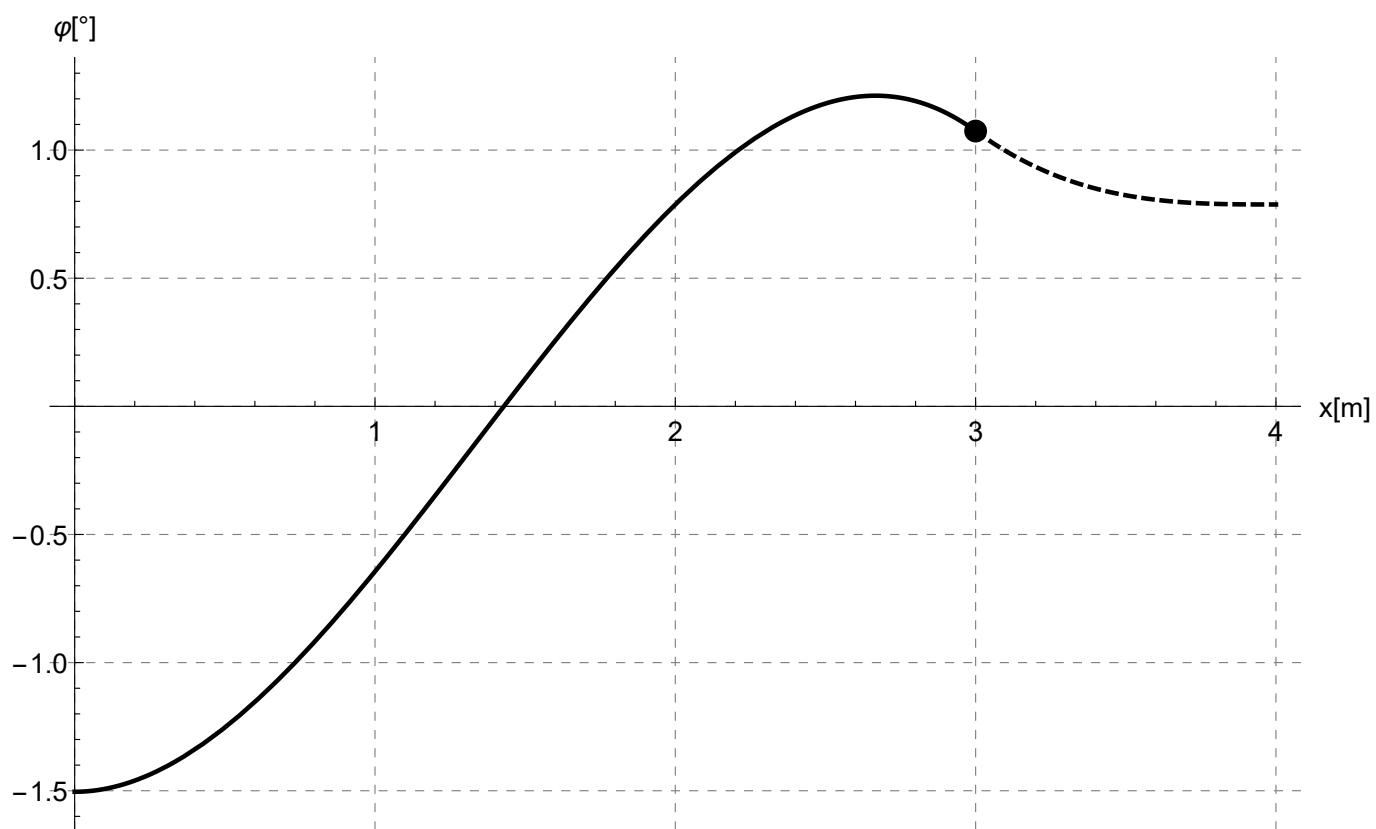
2. ábra. 10.1) szögelfordulás
